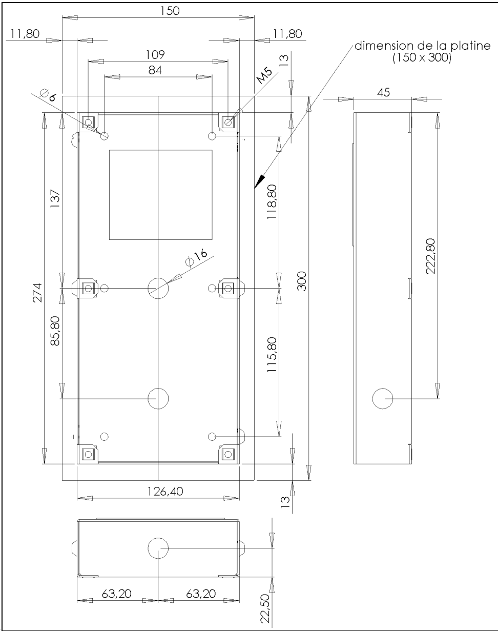
Platine Visio HPIVI3G-V2 : Montage et Encombrement
